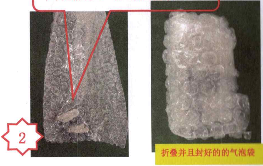
图二，将 2PCS PA2351 如图装入气泡袋，并折叠好。再装入单元格中。（每二个单元格装入一袋）
